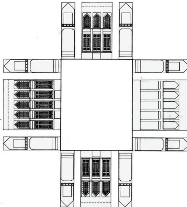
تصویر شماره ۲: شماتیک اتاق‌های سه و پنج دری حیاط بیرونی خانه سنتی، منزل کارزگاه (منبع: موزه آگینه - رسم مجدد از نگارنده)
